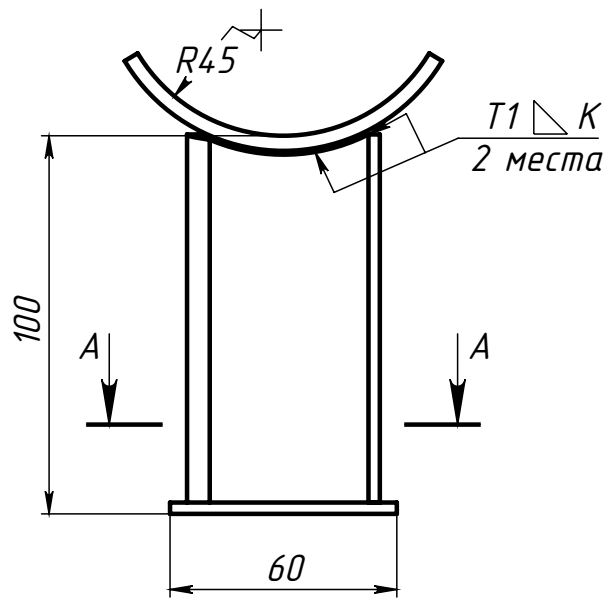
Поз.3 (Ложемент)
